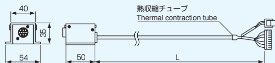
■ 組合せ参考図 Reference Drawing of Combination
