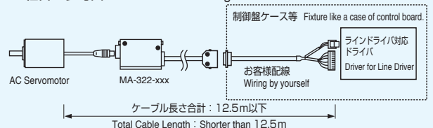
■ 組合せ参考図 Reference Drawing of Combination
