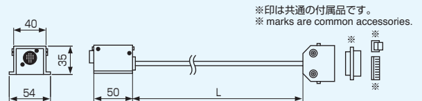
■ 組合せ参考図 Reference Drawing of Combination
